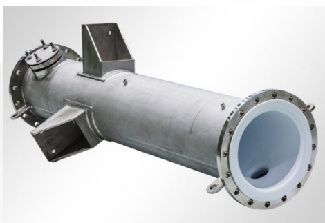
TEFPASS® 塔節
